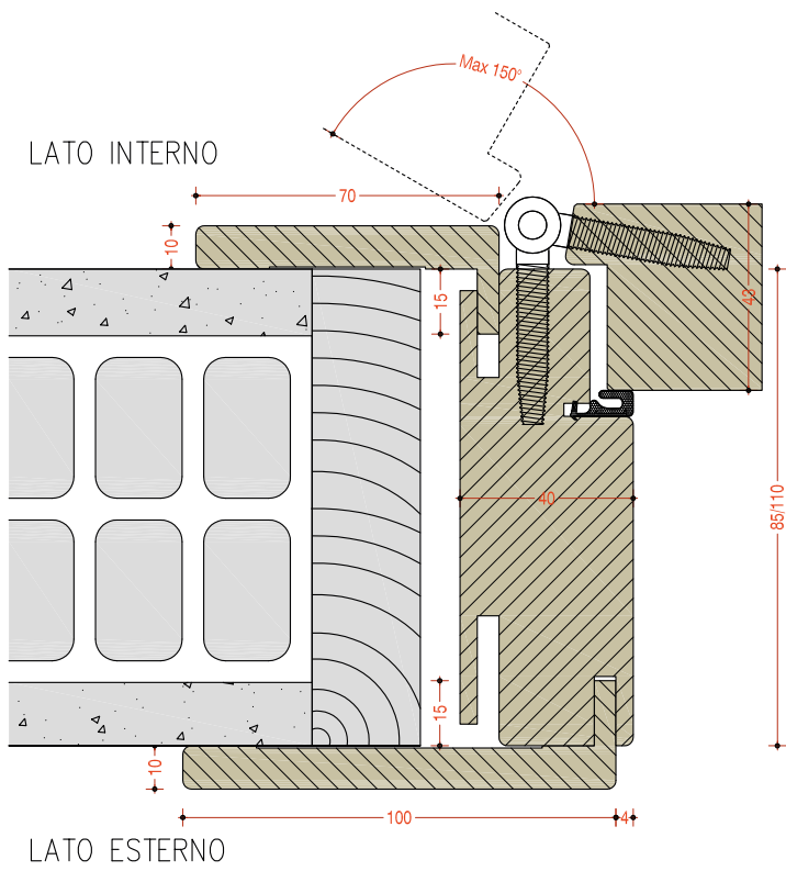
TELAIO STANDARD MOSTRA ESTERNA SEMIFILO
