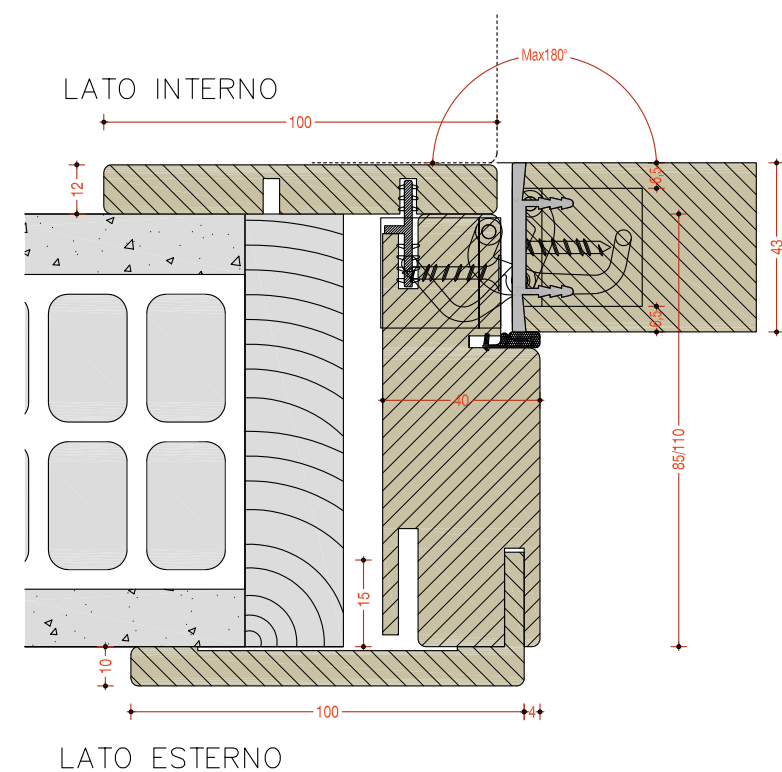
TELAIO ERA - SILVER LINE
