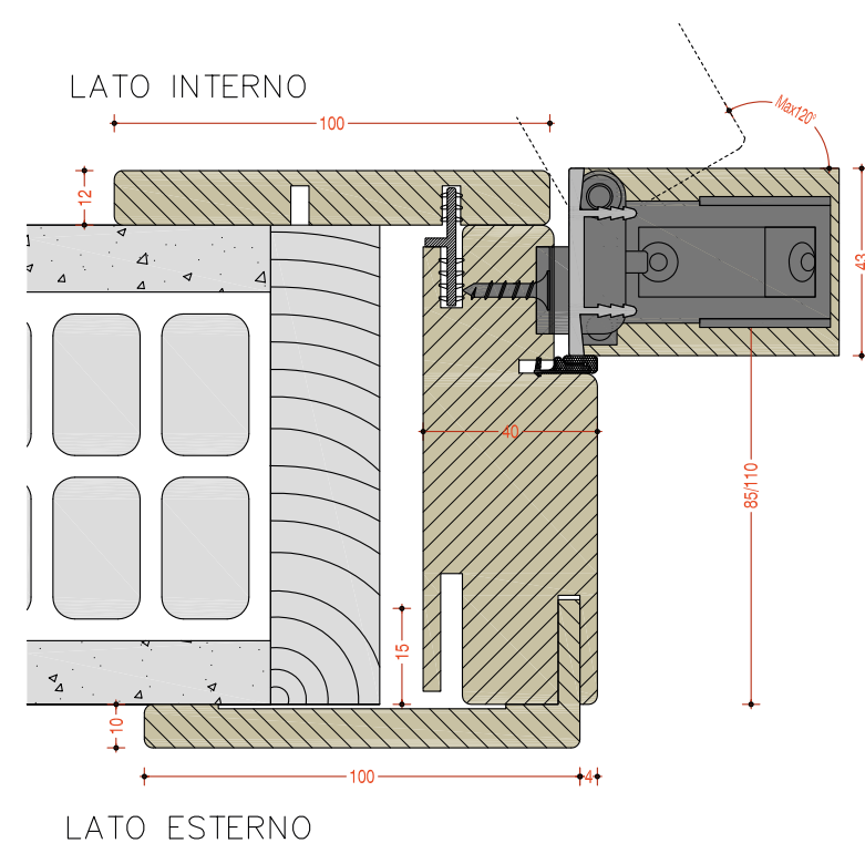
TELAIO EVO - SILVER LINE
