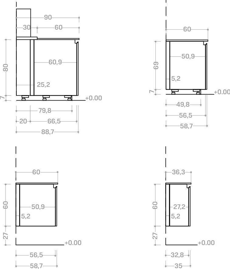
Modulo base con scaffale Medley tipo A-B Base module with Medley type A-B shelf
